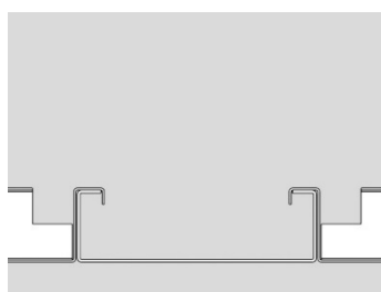
Armstrong nedhængt
