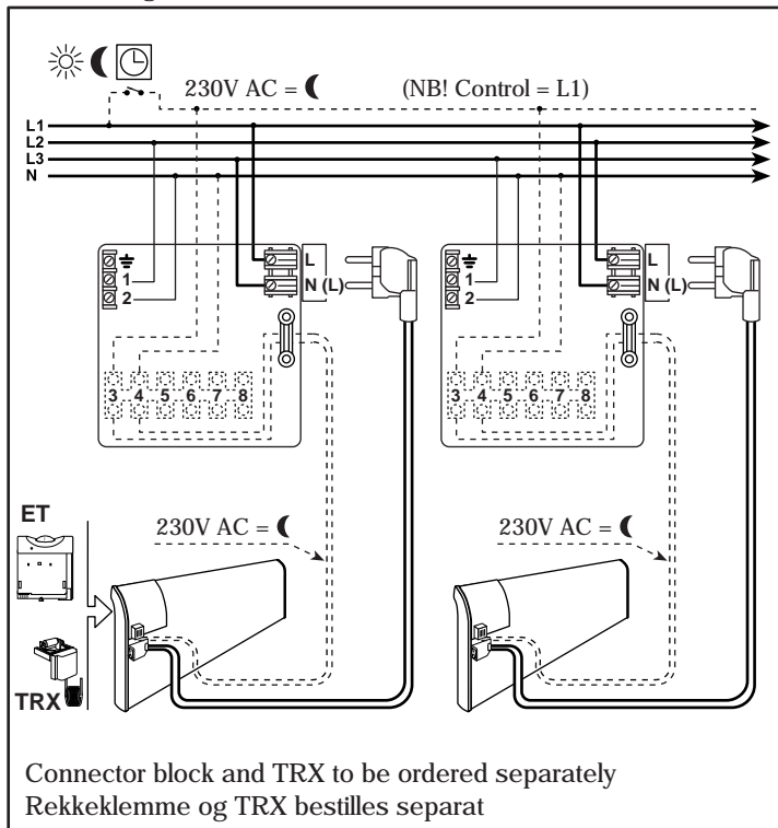
400 volt diagram
