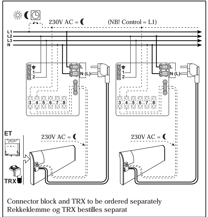
230 volt diagram
