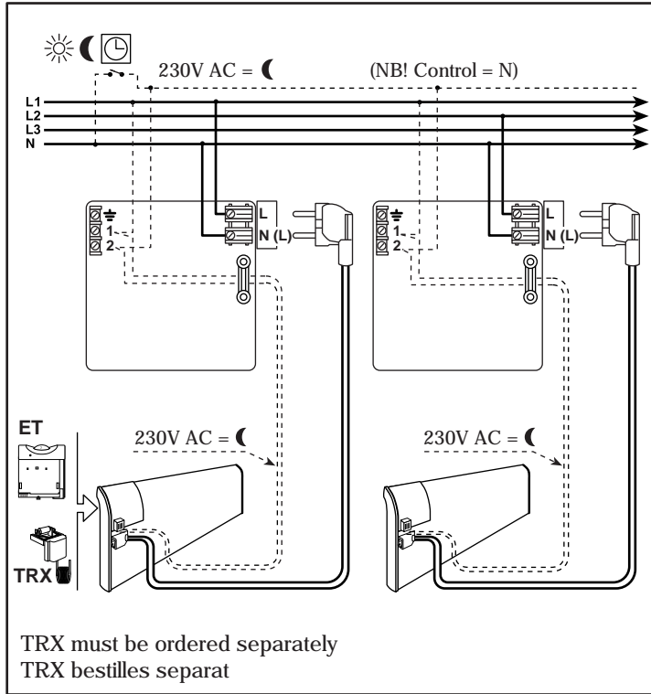
230 volt diagram
